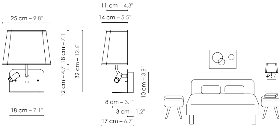
Version droite du lit / Right bedside version Afeusbspotd
