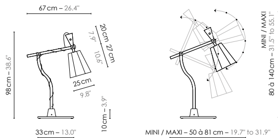
MINI / MAXI – 50 à 81 cm – 19.7" to 31.9" 7 positions de bras et d'abat-jour 7 arm and lampshade positions
